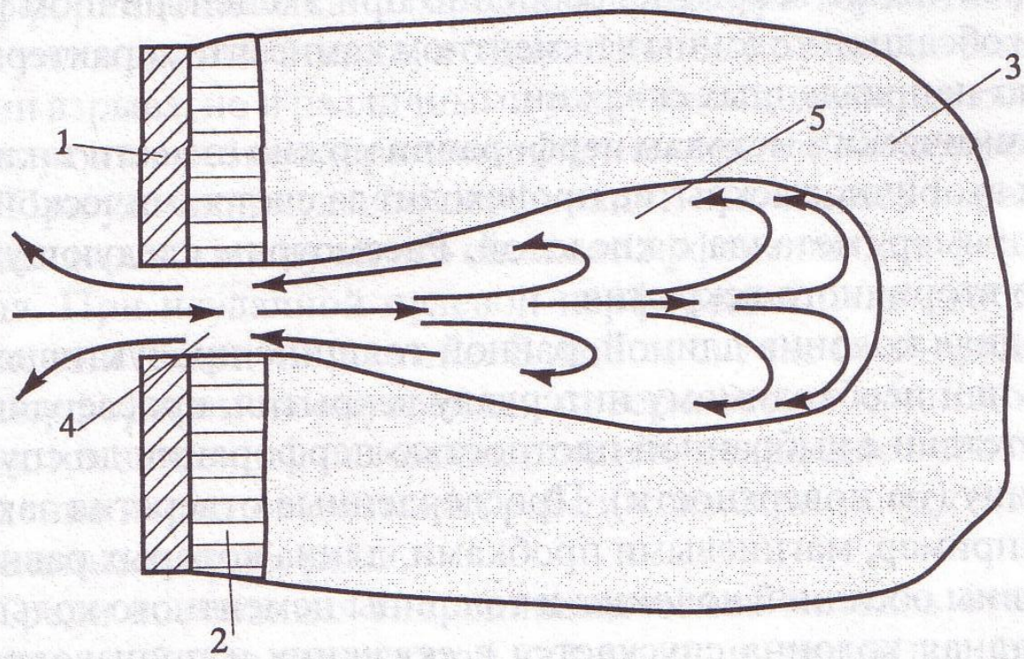
Рис. 1.11. Схема образования грушеобразной каверны в породе при гидropескоструйной перфорации:
