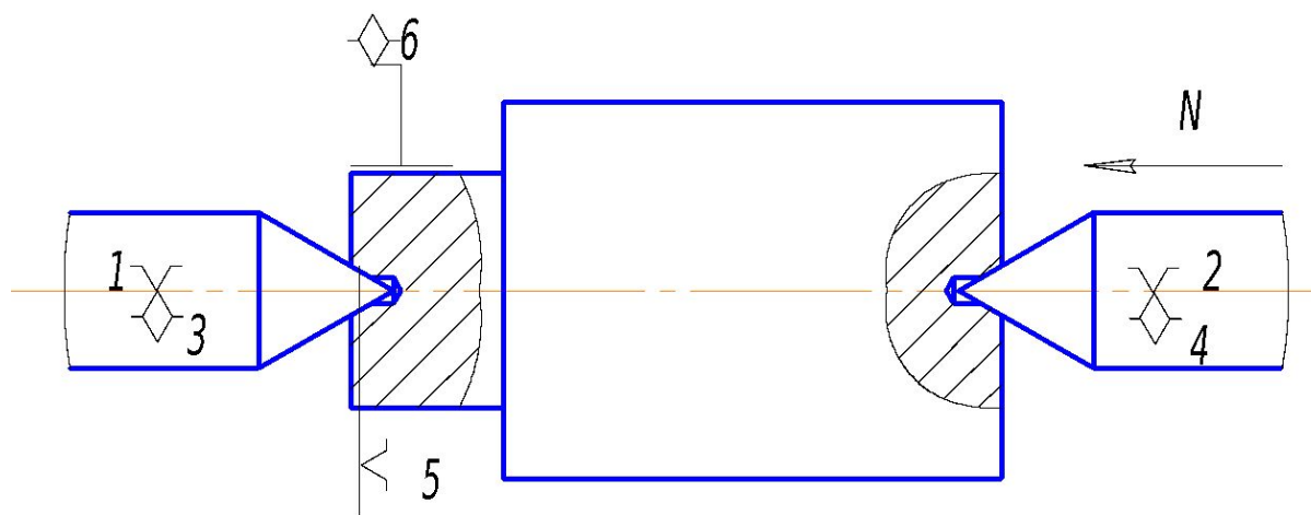
Рис. 5. Агрегат из двойной направляющей и двух опорных
