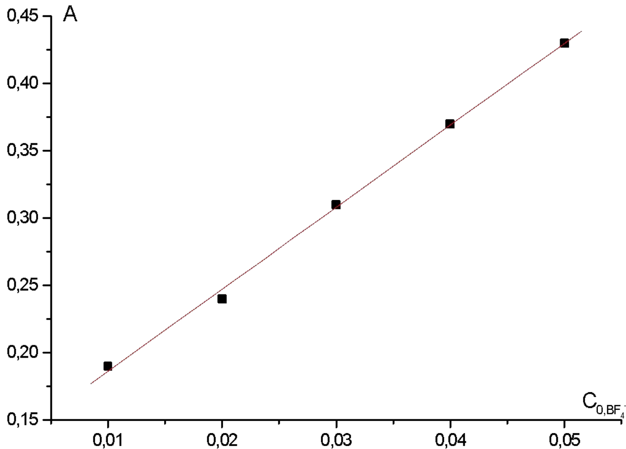
Рис.5.График зависимости оптической плотности от C_{0,BF_4^-} Уравнение прямой: A = 0,13 + 6,10 \cdot C_{0,BF_4^-} ; ( R=0,999 )
