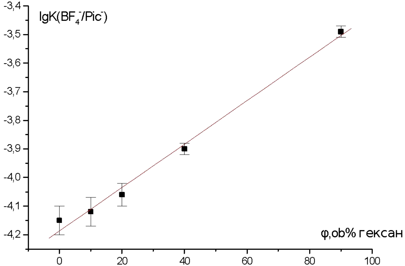
Рис.4. График зависимости \lg K_{\text{Pic}^-}^{\text{BF}_4^-} от \phi , об% гексана. Экстрагент: 1 \cdot 10^{-3} М толуольный раствор пикрата ТНОДА. Уравнение прямой: = -4,187 + 0,008 \cdot \phi ; ( R=0,996 ).
