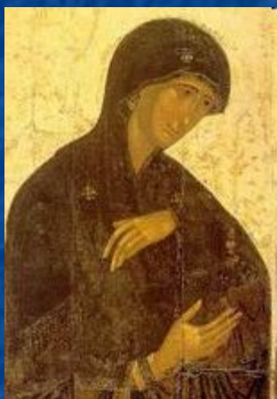
Деисус. Константинополь. 1387-1395
