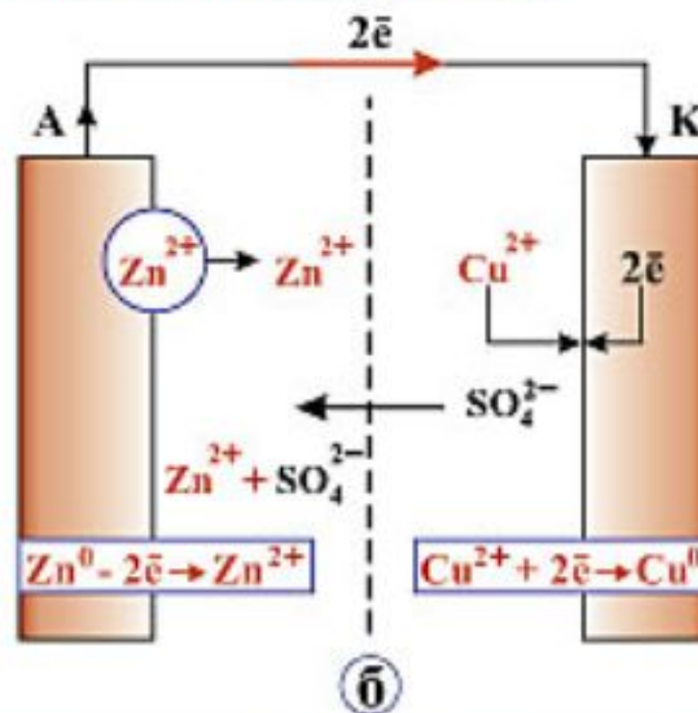
ГАЛЬВАНИЧЕСКИЙ ЭЛЕМЕНТ И СХЕМА ЕГО РАБОТЫ
