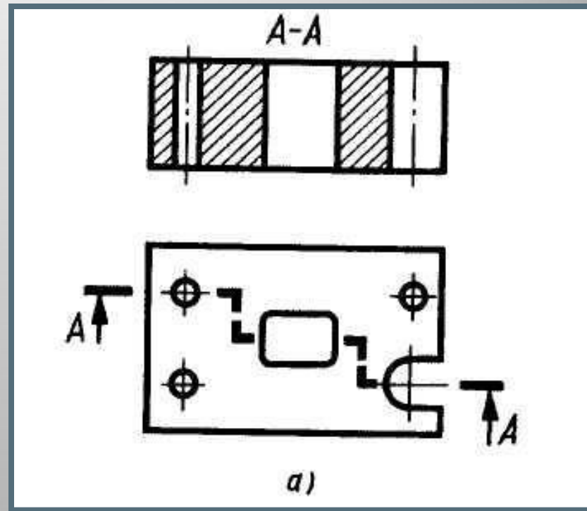
СТУПЕНЧАТЫЙ РАЗРЕЗ
