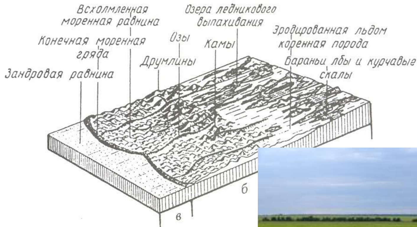
Рис. 123. Схема соотношения ледникового и Области: а — преобладающей ледниковой денудации; б — аккумуляции; в — периглациальной аккумуляции;
