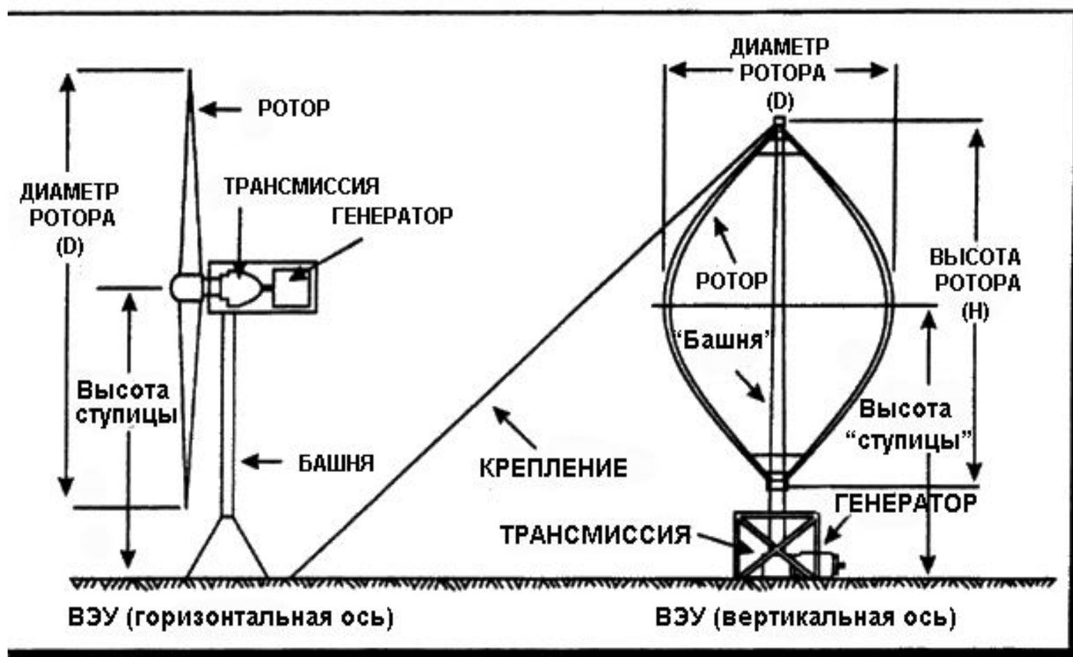
Основные компоненты ВЭУ с горизонтальной и вертикальной осями
