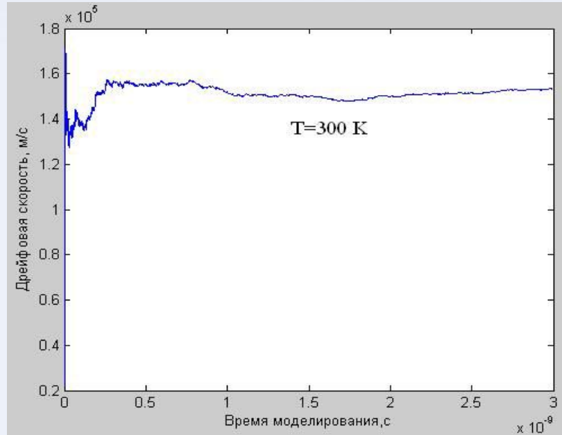
Все механизмы рассеяния
