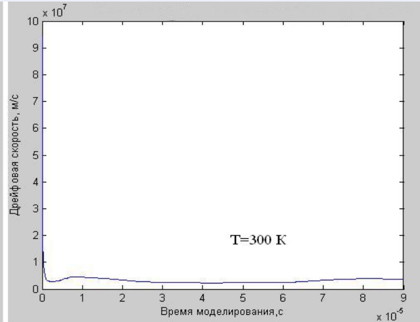
Без рассеяния на полярных оптических фононах
