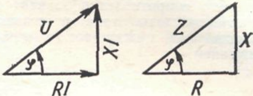
Рис. 6-4. Треугольник напряжений и треугольник сопротивлений при индуктивной нагрузке.
