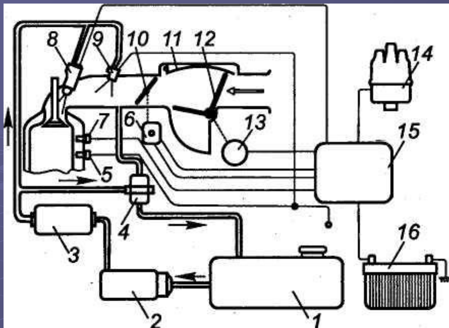
Рис. 11. Схема аппаратуры впрыска бензина «L-Джетроник» фирмы «Роберт Бош»
