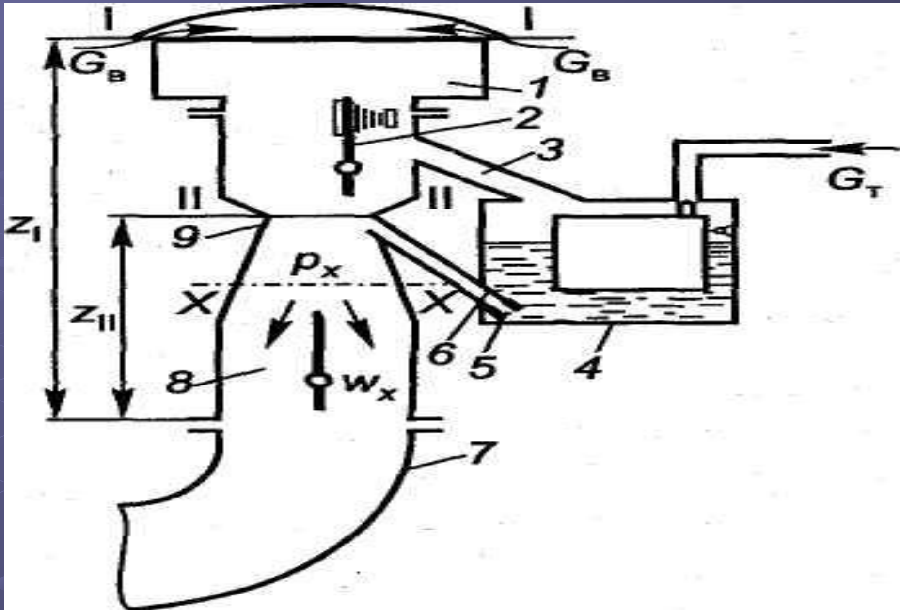
Рис. 1. Схема элементарного карбюратора
