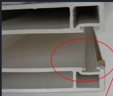
Ламинационная пленка
